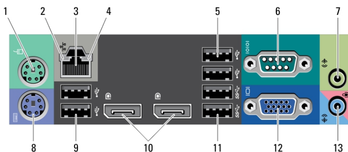
Figur 2. Oversikt over bakpanelet
